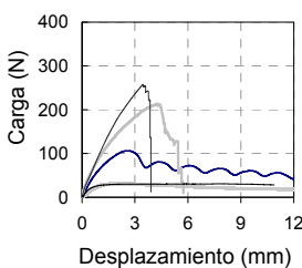
Figura 5. a) Respuestas carga-desplazamiento obtenidas en ensayos de arrancamiento de diferentes fibras; b) variación de la adherencia con la resistencia de la matriz.
