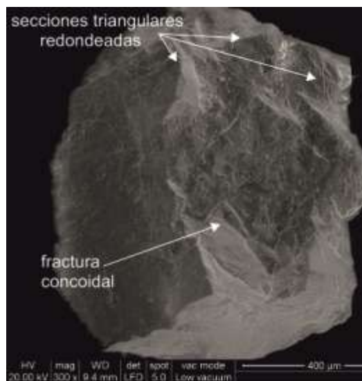
Figura 4: Fotografía obtenida mediante microscopio electrónico de barrido de un cristal de turmalina.
