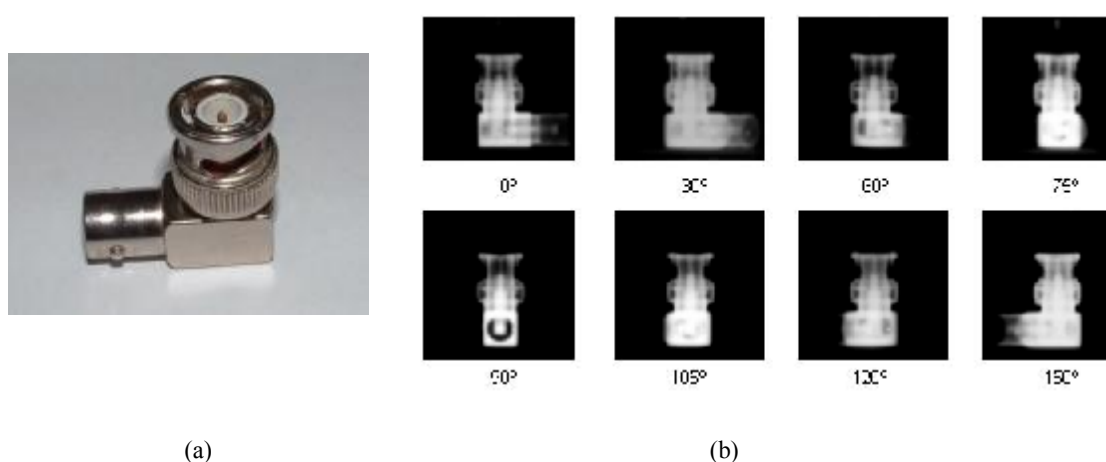
Figura 2. Fotografía de un conector (a) y radiografías tomadas en 8 ángulos diferentes del conector BNC (b).
