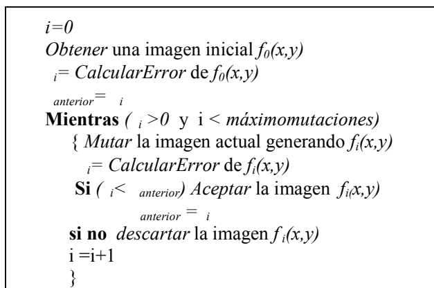
Figura 3. Esquema básico del algoritmo Monte Carlo
