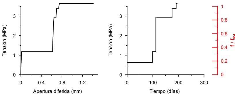
Figura 3- Viga D1. Curvas Tensión- Apertura de fisura y Tensión-Tiempo ( f_{R4} = 3,0 MPa).
