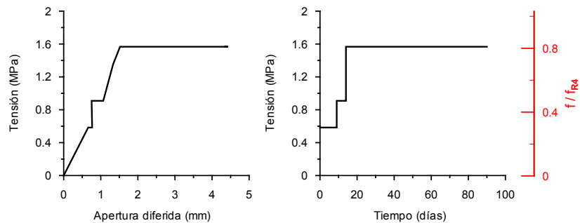
Figura 2 - Viga A1. Curvas Tensión- Apertura de fisura y Tensión-Tiempo ( f_{R4} = 1,9 MPa).
