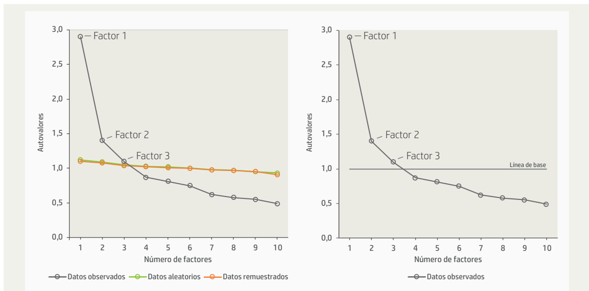
Figura 1. Valores de los componentes principales de los datos, según análisis paralelo y de autovalores de las preguntas del índice de capacidad para el trabajo. Bahía, Brasil, 2011-2012.
