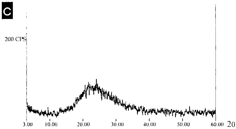
Difractograma de rayos X de perlita expandida natural. Se observa que se trata de material amorfo.
