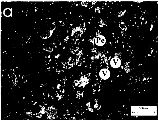
Fracción 50-100 Pe = Perlita V = Vidrio natural sin expansión
