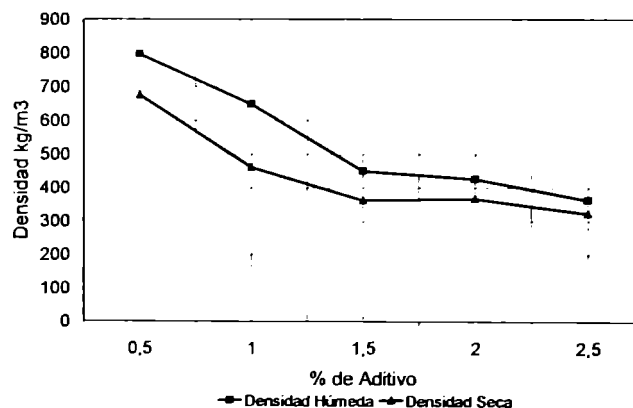
Graf. 1: Densidad fresca y aparente vs. Cantidad de aditivo
