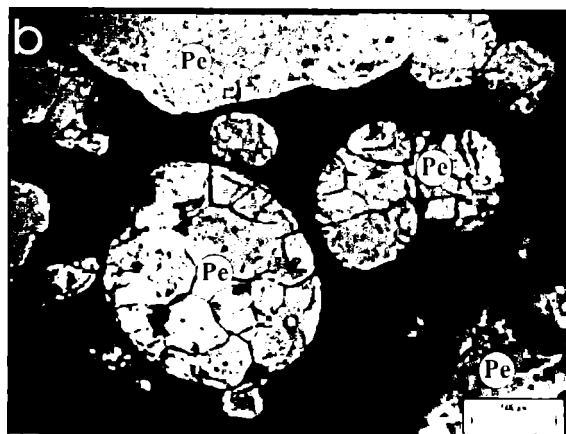
Distintas texturas y morfología de la perlita (Pe) en el mortero.
