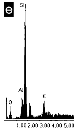
EDAX de la imagen observada en 1 c.
