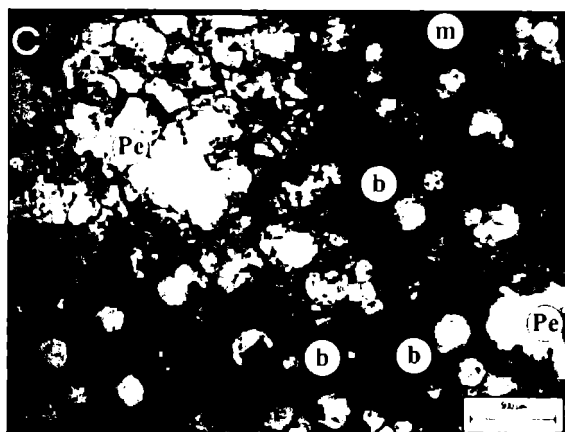
Contacto neto de perlita (Pe) – mortero (m) Abundante desarrollo de burbujas de aire (b)
