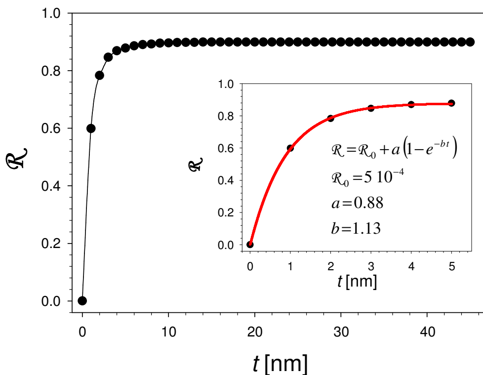
Fig VI.2.1.2.1: Reflectividad diferencial calculada \mathcal{R} en función del espesor del óxido de plata t para una onda polarizada p. El inset muestra una ampliación de la curva en el rango de espesores de óxido de 0 - 5 nanómetros
