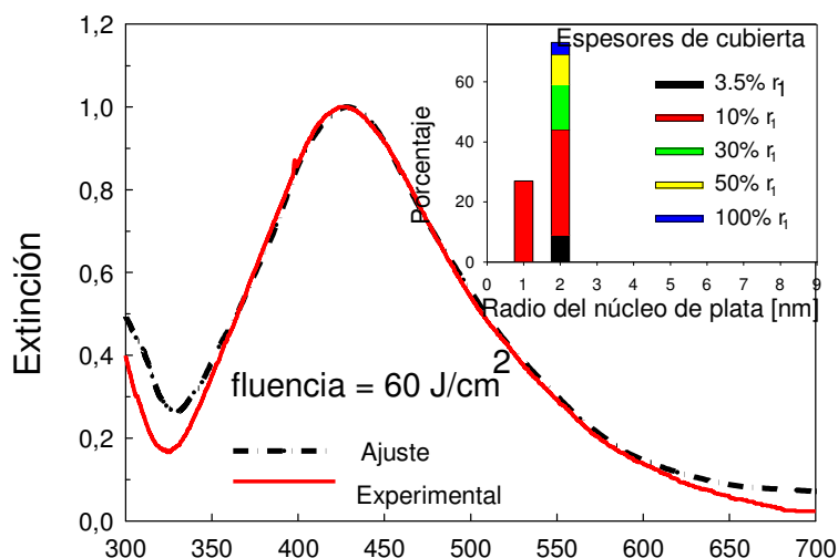
Fig. V.5.1.1: Espectro experimental de extinción (línea llena) y ajuste teórico (línea de puntos y rayas) para Nps de plata en agua irradiadas con fluencias de 60 J/cm 2 . El inserto muestra la distribución de tamaño usada para el ajuste.
