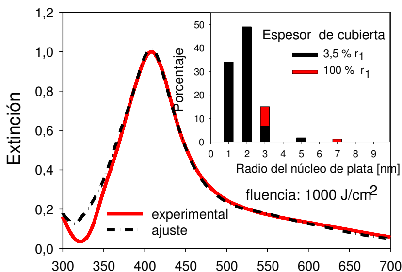
Fig. V.5.1.5: Espectro experimental de extinción (de línea llena) y ajuste teórico (línea de puntos y rayas) para Nps de plata en agua en 1000 \text{ J/cm}^2 fluencia. El inserto muestra la distribución de tamaño utilizada para el ajuste.
