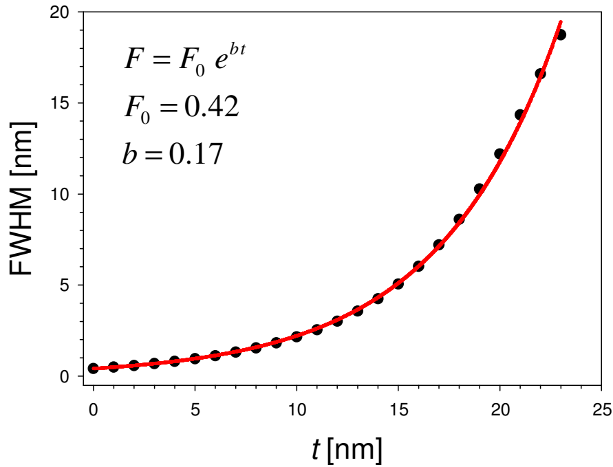
Figura VI.2.1.3.1: FWHM (indicado como F en la ecuación del inset) de la curva de reflectancia calculada para una onda polarizada p para diferentes espesores t de óxido de plata \text{Ag}_2\text{O} crecidos sobre una capa de plata.
