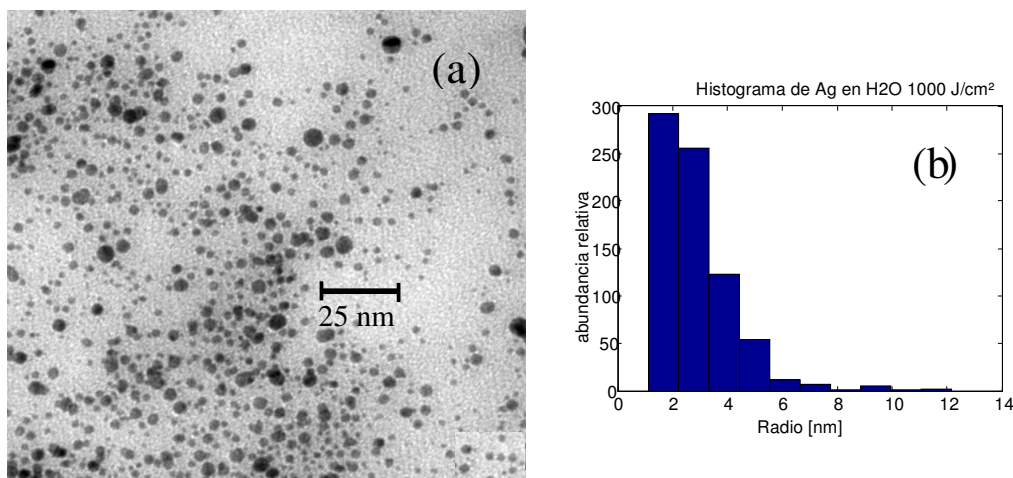
Fig. V.5.2.1: (a) Imagen TEM y (b) histograma correspondiente a la muestra de Nps de plata sumergida en el agua, fabricada con una fluencia alta (1000 J/cm 2 ).
