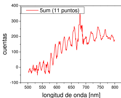
Fig III.2.1.d. Espectro reducido correspondiente a partículas de 5\mu\text{m} al que se le aplicó un promedio de medias móviles de 11 puntos adyacentes.
