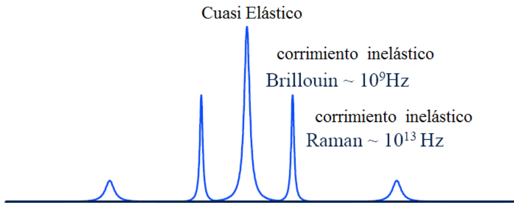
Fig.I.2.4.2 Interpretación esquemática del espectro para scattering cuasi elástico y corrimiento Raman .
