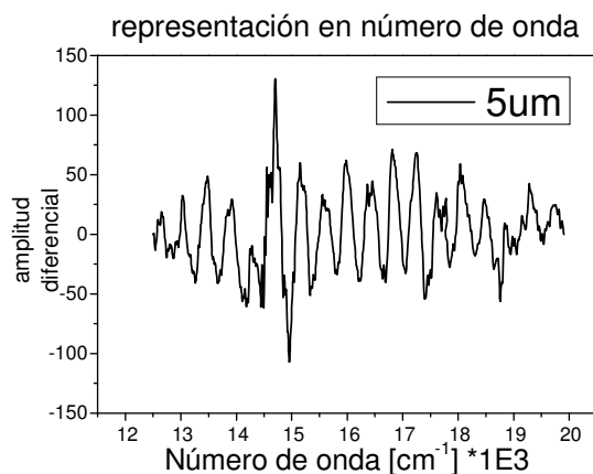
Fig III.2.3.1 Representación del espectro reducido en \text{cm}^{-1} (Escala recíproca) correspondiente a partículas de 5\mu\text{m} .
