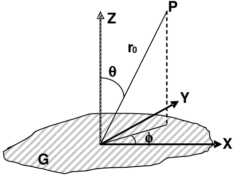
Fig.II.2.4.2.1 Representación del punto de observación P dispuesto para el cálculo de la radiación dispersada por la superficie G.
