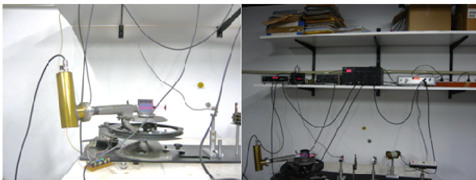
Fig I.3.8.1 Arriba, esquema de un sistema detector de intensidad angular. Abajo a la izquierda detalle de la celda donde puede apreciarse el haz de He Ne atravesando la solución de partículas y disposición de los instrumentos de medida y otros dispositivos (Centro de Investigaciones Ópticas CIC BA CONICET).
