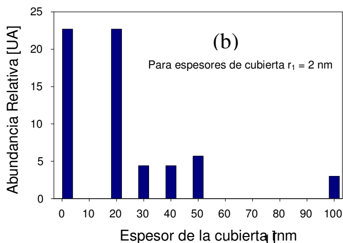
Fig. V.5.2.2: (a) Espectro experimental de rayas) para Nps de Ag en etanol irradiadas con una fluencia de 1000 \text{ J/cm}^2 . El inserto muestra la distribución de tamaños correspondientes al ajuste. (b) Histograma de abundancia relativa de espesores de cubiertas para núcleos de 2 nm.
