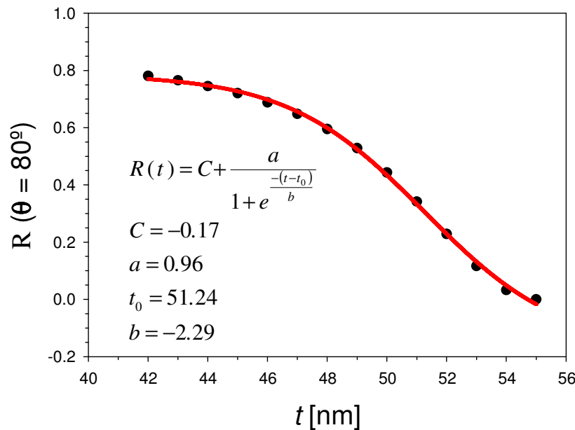
Fig. VI.2.2.2.1: Reflectividad R en \theta = 80^\circ en función del espesor de \text{Ag}_2\text{O} para una onda polarizada
