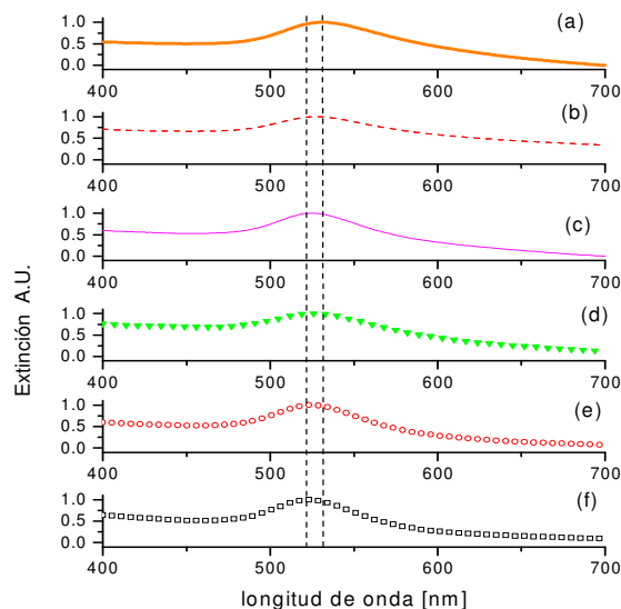
Fig. IV.3.1.2 Espectros normalizados de extinción que corresponden a Nps oro obtenidas con fluencias de: 416 (b), 342 (c), 291 (d), 256 (e) y 0.8 (f), \text{J}/\text{cm}^2 . También se incluye a efectos de comparar, el espectro de extinción de la solución inicial (a).
