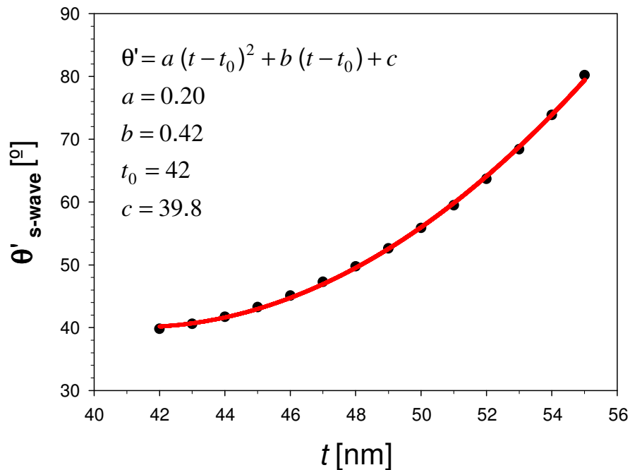
Fig. VI.2.2.1.1: Mínimo de la reflectividad ( \theta' ) en función del espesor t \text{Ag}_2\text{O} para una onda polarizada s . Los círculos corresponden a los valores calculados y la línea sólida al ajuste cuadrático.
