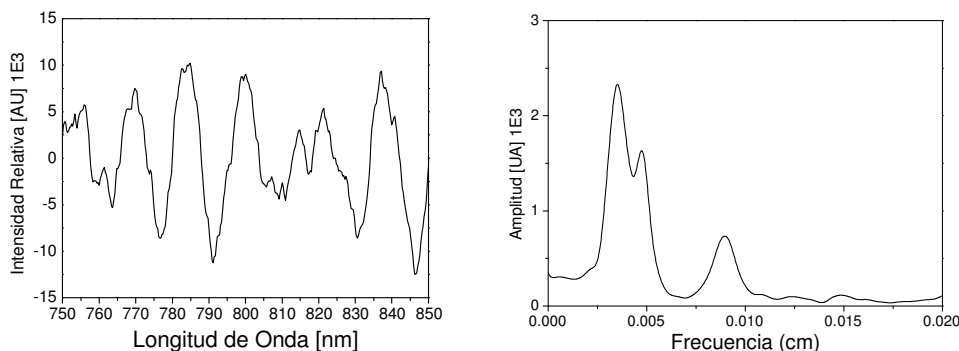
Fig III.5.3.1 Espectro en el rango IR obtenido para una mezcla de partículas de 8 10 y 20 \mu\text{m} de diámetro y su TF. Puede observarse la aparición de picos correspondientes a diferentes diámetros presentes en la muestra.
