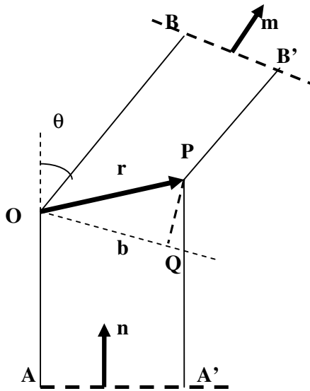
Fig II.2.4.1.1 Geometría del scattering de Rayleigh Gans donde: \mathbf{n} es la dirección de incidencia, \mathbf{m} dirección de scattering, \mathbf{r} pertenece al plano formado por \mathbf{m} y \mathbf{n}
