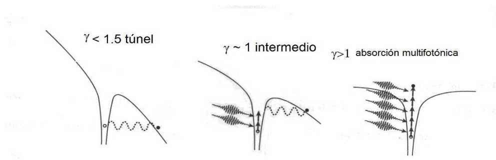
Fig IV.2.2.1: Esquema de los mecanismos de ionización por supresión de barrera o túnel y multifotónicos.[63][64].
