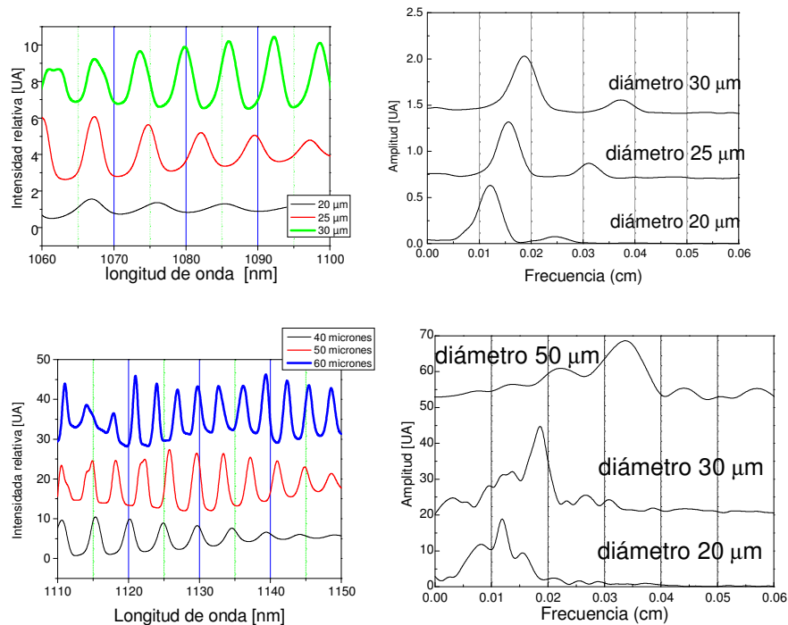
Fig III.5.2.1. Espectros de partículas de 20, 30 y 50 \mu\text{m} de diámetro en el rango NIR y sus respectivas TF en el rango en que presentan un pico
