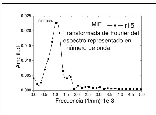
Fig III.2.4.4. Espectro total obtenido de la representación en \text{nm}^{-1} * 1\text{E}7 correspondiente a partículas de 1.5\mu\text{m} de radio.
