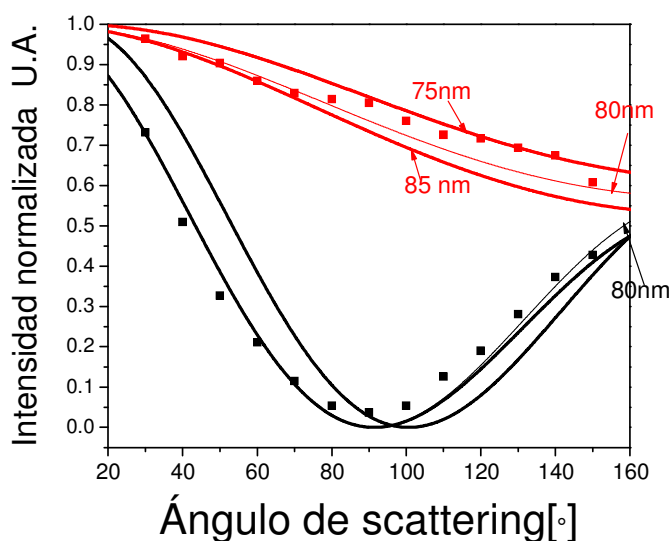
Fig. I.3.8.2 Ajuste de medidas de intensidad angular En líneas gruesas curvas extremas 85 y 75 nm. La línea delgada representa el mejor ajuste por teoría de Mie. En puntos cuadrados registros experimentales. Se hace notar que esta figura es una versión en coordenadas cartesianas de la figura I.3.7.2
