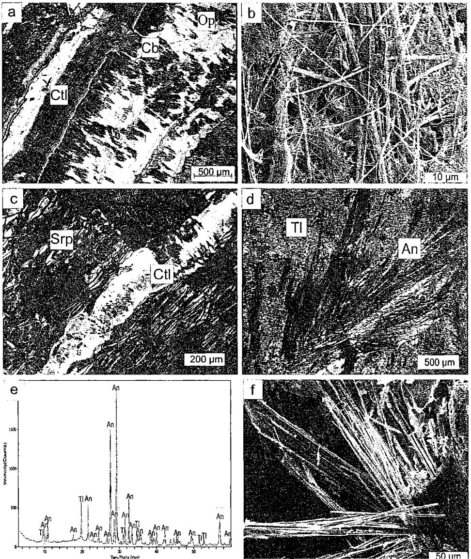
Figura 3: a) Venillas subparalelas con un bandeamiento irregular, donde el crisotilo cristalizó en forma transversa (mina La Bélgica), b) Detalle de las fibras observadas con MEB, c) Antigorita y lizardita atravesada por venillas discordantes de crisotilo (cantera Vitale), d) Anfíbol con morfología acicular asbestiforme asociado a talco (mina La Adita), e) Difractometría de rayos X de antofilita y talco en la zona de venillas de mina La Isla, f) Morfología fibrosa, acicular de los minerales con un gran desarrollo cristalino (MEB, mina Mauro).
