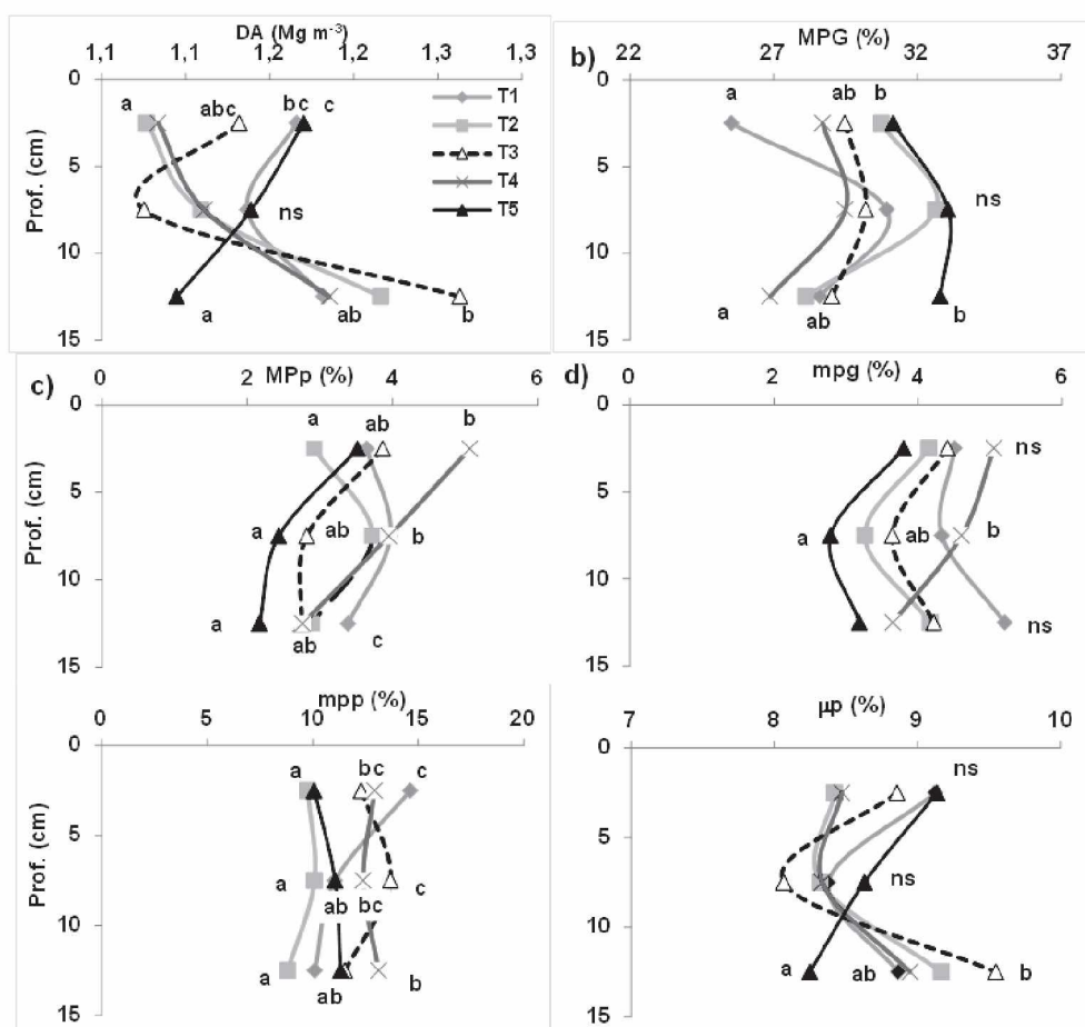
Figura 1: a, Densidad aparente (DA); b, macroporos grandes (MPG); c, macroporos pequeños (MPp); d, mesoporos grandes (mpg); e, mesoporos pequeños (mpp); f, microporos ( \mu p ) del suelo con diferentes enmiendas. T1: Testigo, T2: Bioorganutsa, T3: compost de cebolla-estiercol, T4: lombricompost, T5: Azospirillum.
