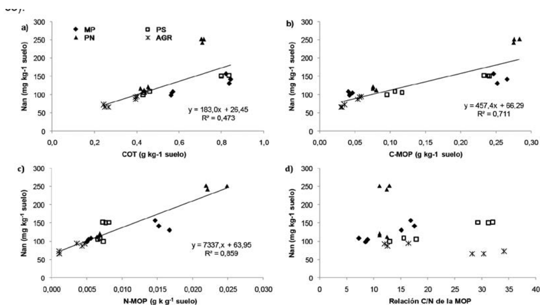
Figura 3: Relación entre nitrógeno incubado en anaerobiosis (Nan) y carbono orgánico total (COT) (a), carbono en la fracción MOP (C-MOP) (b), nitrógeno en la fracción MOP (N-MOP) (c) y relación C/N de la fracción MOP (d).
