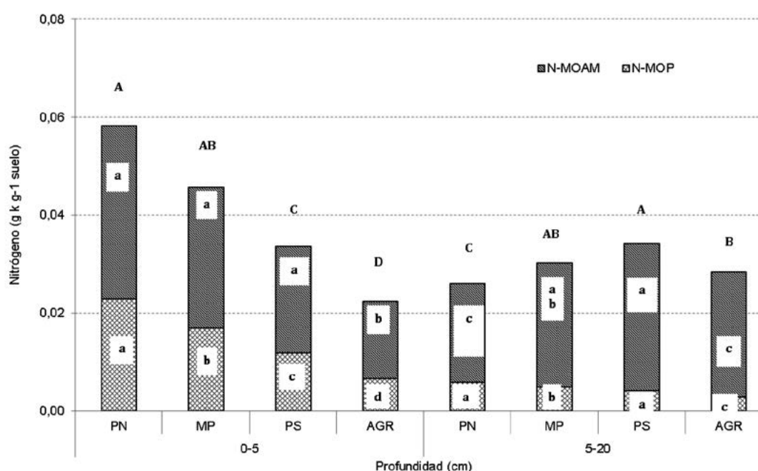
Figura 2: Nitrógeno en las fracciones MOP y MOAM, en sitios bajo pastizal natural (PN), monte de pinos (MP), pastizal secundario (PS) y agricultura (AGR) a dos profundidades. La suma de N-MOP y N-MOAM representa el Nt.
