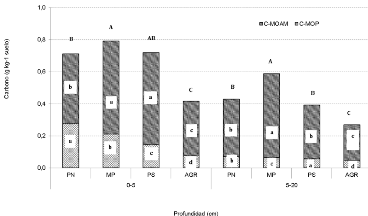
Figura 1: Carbono en las fracciones MOP y MOAM en sitios bajo pastizal natural (PN), monte de pinos (MP), pastizal secundario (PS) y agricultura (AGR) a dos profundidades. La suma de C-MOP y C-MOAM representa el COT.
