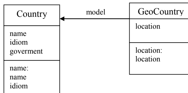
Figura 1: El decorador GeoCountry, decora a la clase conceptual Country
