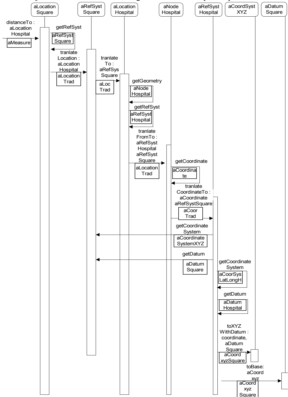
Figura 6. Diagrama de interacción, asumiendo que el sistema de referencias en común es el del objeto geoSquare
