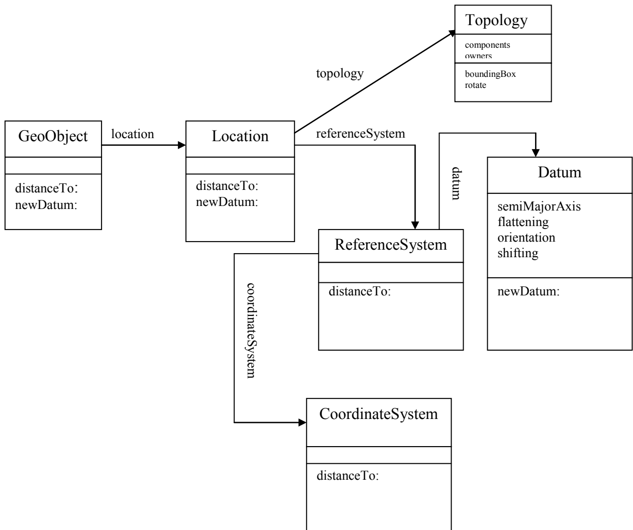
Figura 3: Las clases Datum y Coordinate System contempladas en el modelo
