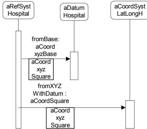
Figura 7. Conversión desde coordenadas base a coordenadas de destino
