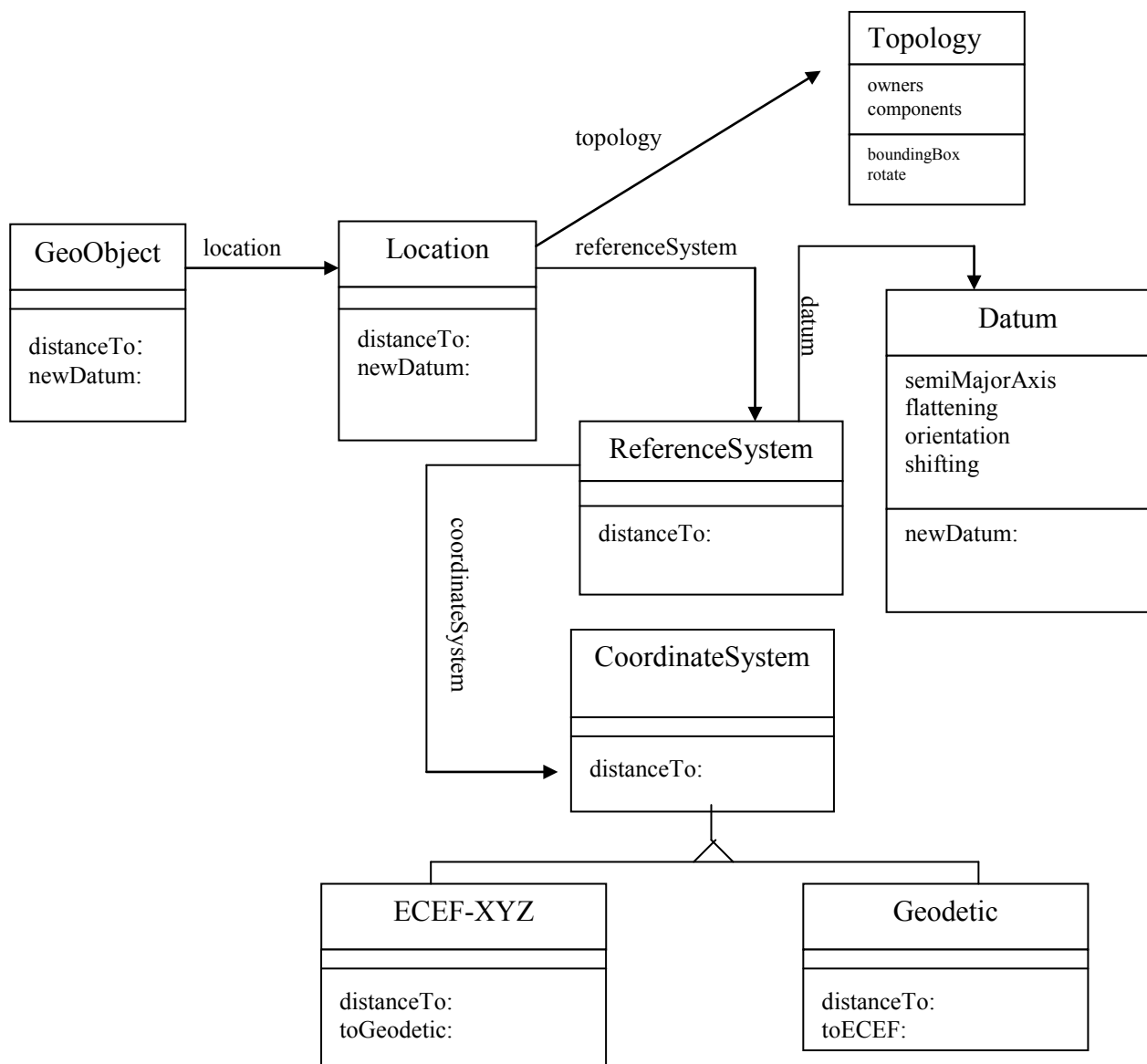
Figura 4: Subclasificación de la clase CoordinateSystem
