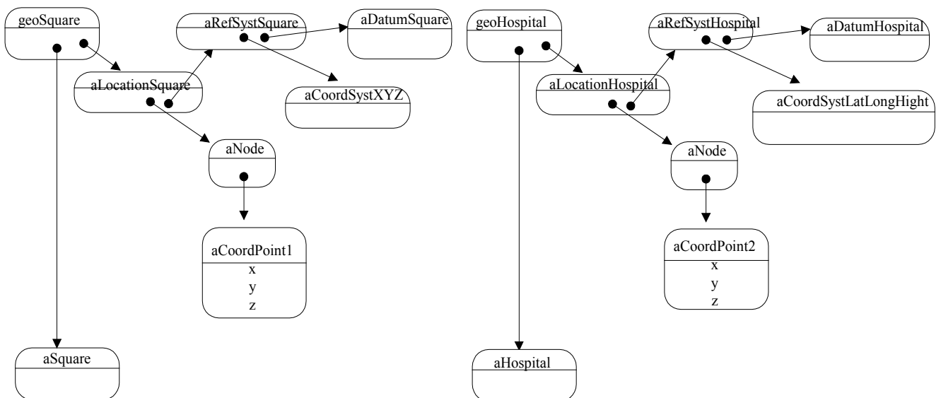
Figura 5. Diagrama de objetos. Relaciones entre las instancias
