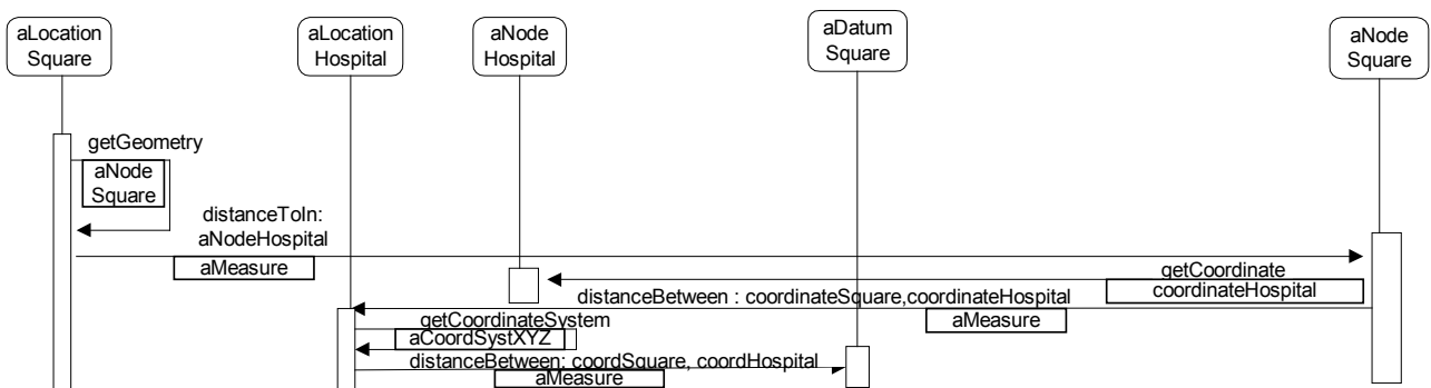
Figura 8. Cálculo de distancia entre dos Location expresadas en el mismo Sistema de Referencias.
