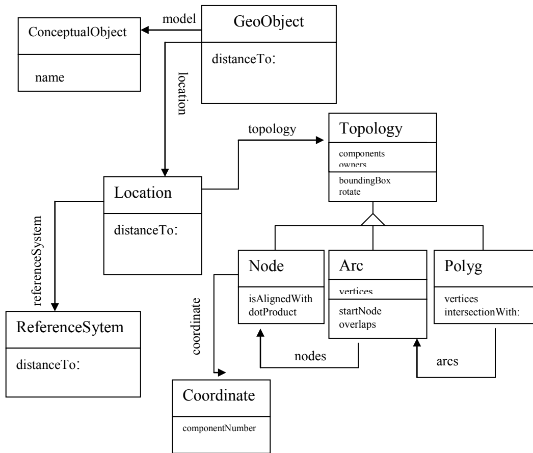
Figura 2: Relación entre el objeto conceptual (ConceptualObject), el geográfico (GeoObject) y la Location
