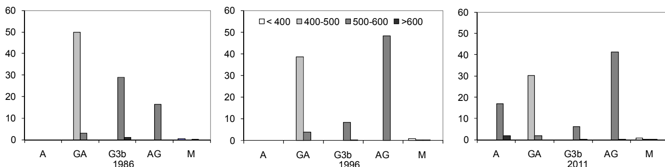
Figura 4. Clases de rendimiento hídrico ( \text{m}^3.\text{píxel}^{-1} ) en porcentaje de ocupación según escenarios de uso del suelo en la cuenca del Arroyo Napaleoufú.
