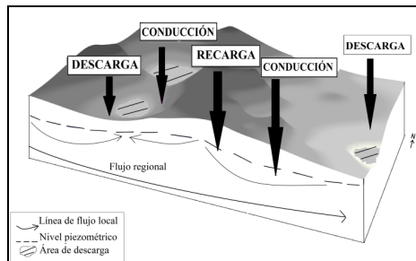
Figura 1: Esquema general del flujo subterráneo. Croquis fuera de escala.
