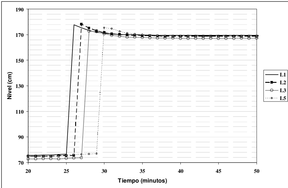
Figura 3. Variaciones de nivel de los instrumentos en el momento de su inmersión en el agua.
