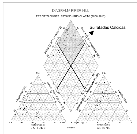
Figura 5. Tipo geoquímico de precipitaciones.
