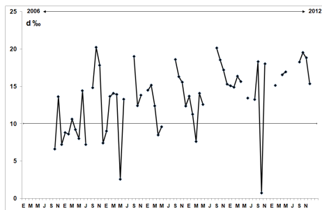
Figura 11. d (‰) de la precipitación. Período 2006-2012.
