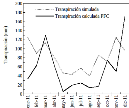
Figura 4. Transpiración mensual calculada mediante plano de flujo cero (PFC) y simulada.
