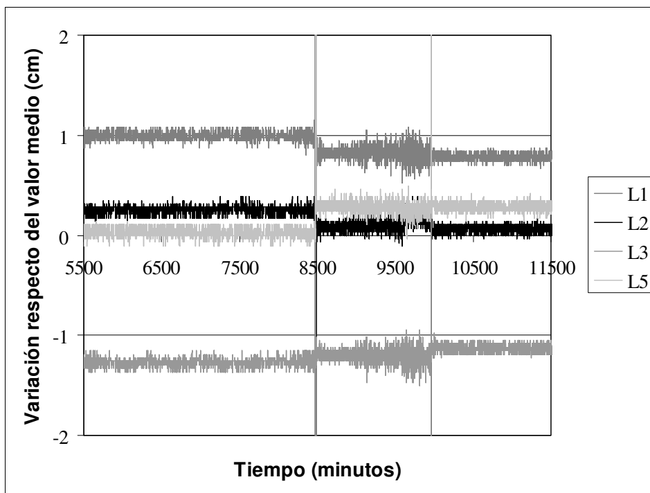
Figura 2. Curvas del valor medido al que se le ha restado el valor medio de la presión atmosférica. Se observa que el ruido de fondo tiene un valor similar a la resolución indicada por el fabricante.
