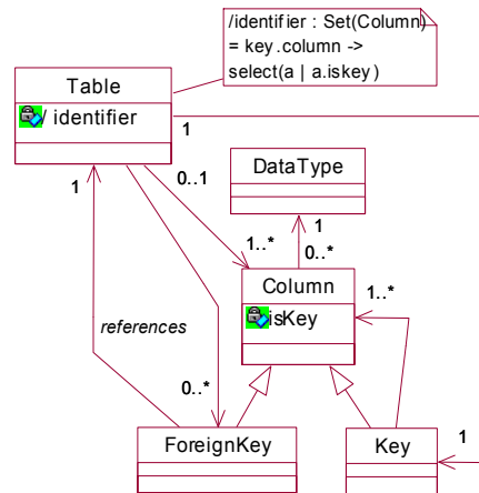
Figura 8. Metamodelo Relacional
