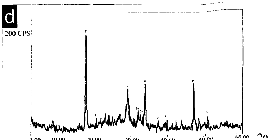
Fractograma de rayos X del hormigón en perlita = Portlandita = Calcita = Silicato de calcio
