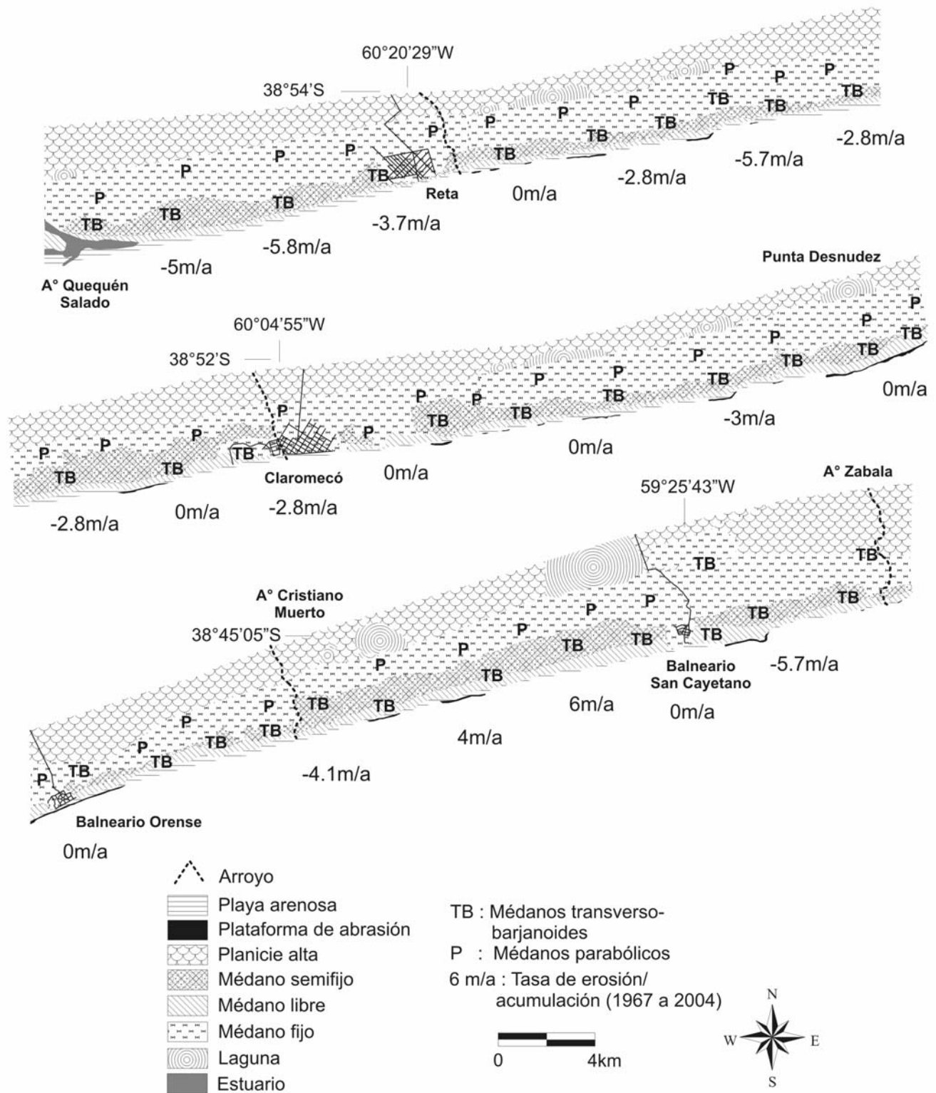
Figura 3: Mapa geomorfológico del área costera.
