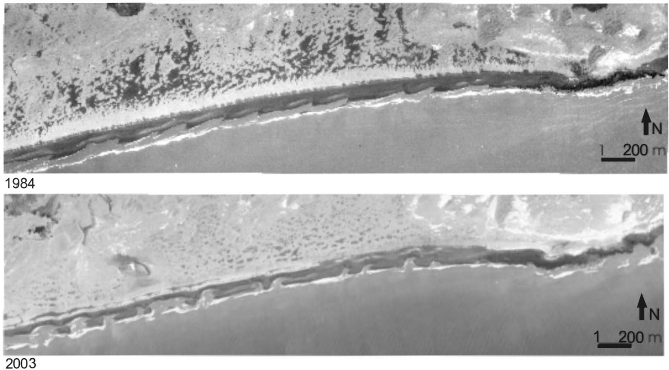
Figura 5: Barras y canales intermareales oblicuos a la costa. Años 1984 y 2003.
