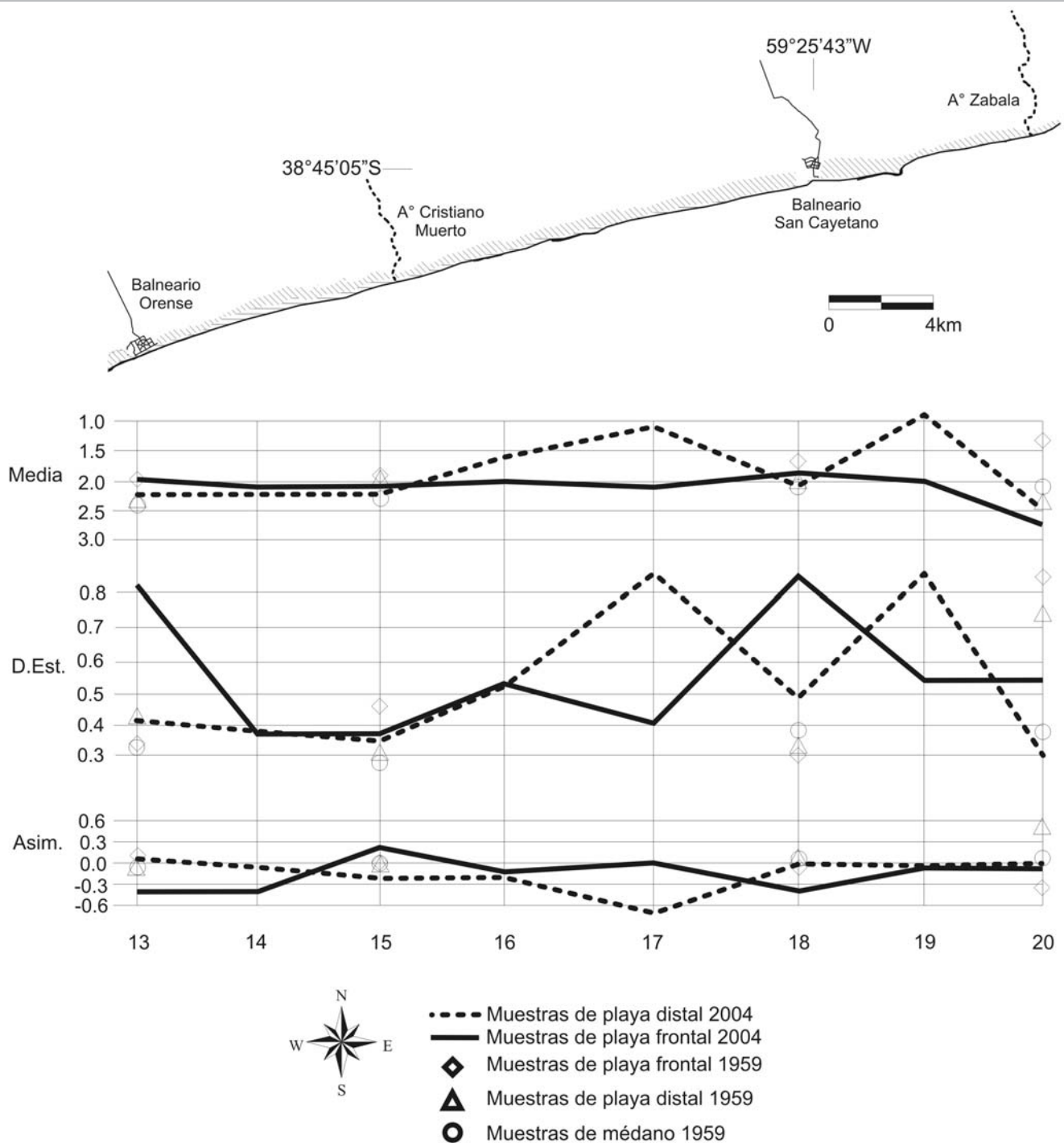
Figura 8: Parámetros sedimentológicos y variaciones de la línea de costa del sector Orense - Arroyo Zabala.
