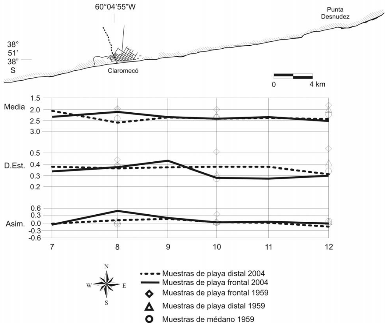
Figura 7: Parámetros sedimentológicos y variaciones de la línea de costa del sector Claromecó - Punta Desnudez.
