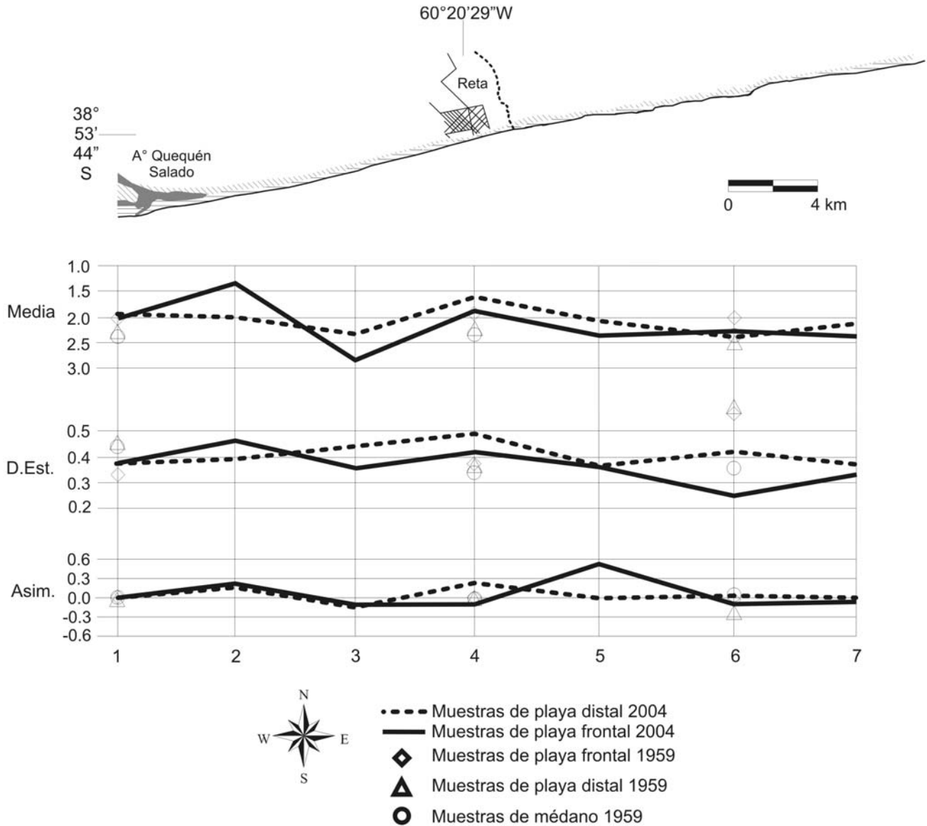
Figura 6: Parámetros sedimentológicos y variaciones de la línea de costa del sector Arroyo Quequén Salado - Claromecú.
