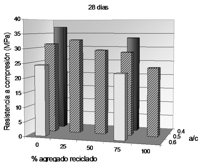
Figura 3. Resistencias a compresión determinadas en hormigones convencionales y reciclados
