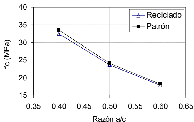
Figura 2. Relación entre la resistencia a compresión ( f_c ) y la razón agua-cemento
