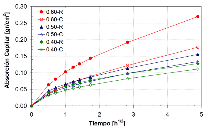
Figura 4. Absorción capilar de hormigones convencionales y reciclados
