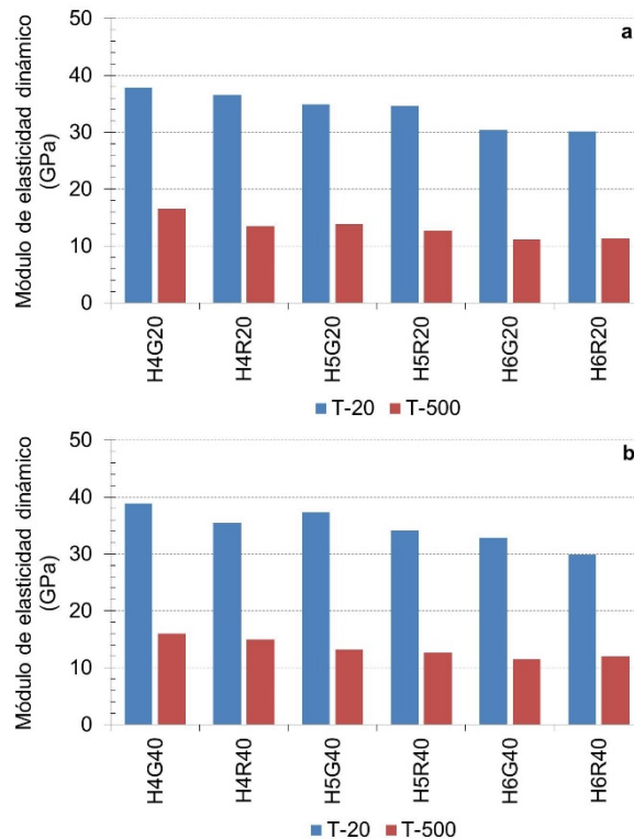
Figura 11. Módulo de elasticidad dinámico de hormigones convencionales y reciclados con 20 y 40 % de AFR, antes y luego de la exposición a alta temperatura
