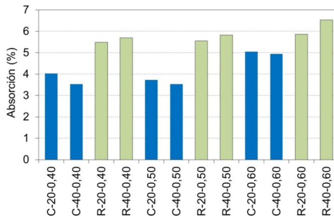
Figura 9. Absorción de agua de hormigones de distintos niveles resistentes, elaborados con 20 y 40 % de AFR
