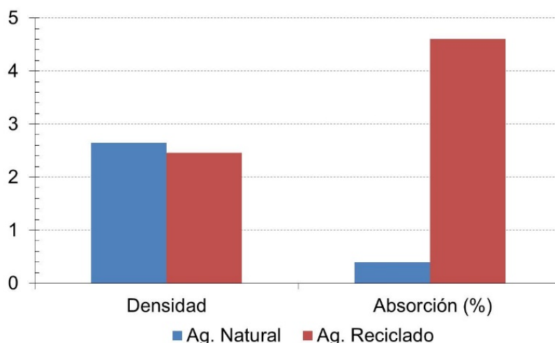
Figura 1. Densidad y absorción de agregados gruesos natural y reciclado
