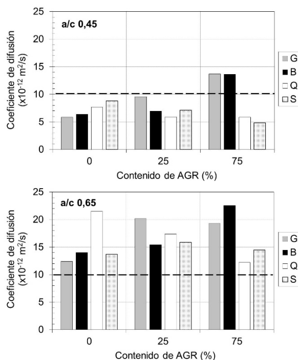
Figura 5. Difusión de cloruro en hormigones convencionales y reciclados con distintos agregados naturales
