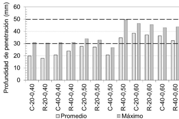
Figura 10. Penetración de agua a presión de hormigones convencionales y reciclados con 20 y 40 % de AFR
