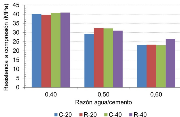
Figura 8. Resistencia a compresión de hormigones de distinta relación a/c, elaborados con 20 y 40 % de AFR
