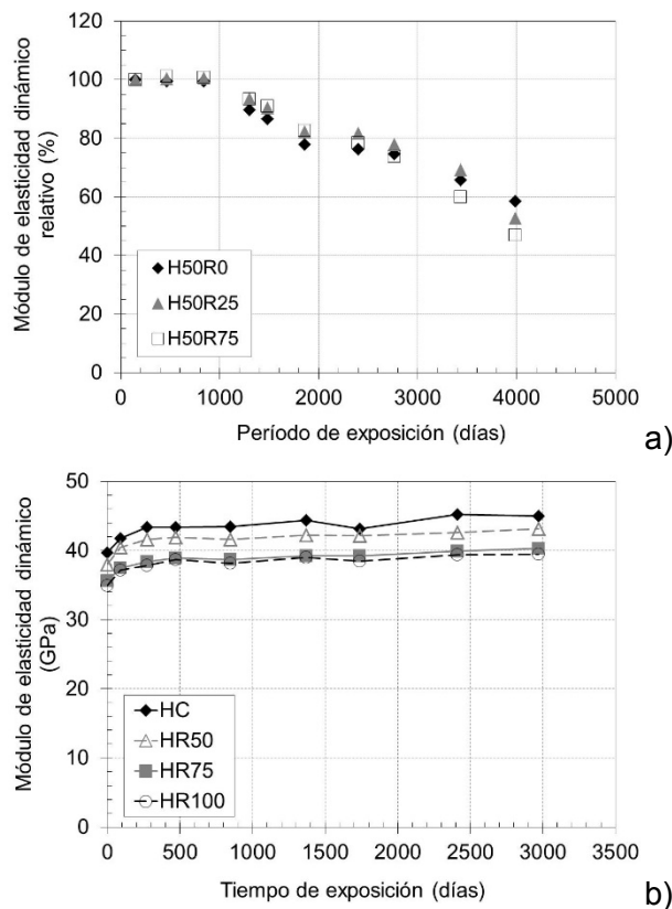
Figura 6. Variación del módulo dinámico de hormigones reciclados expuestos en suelo con sulfato
