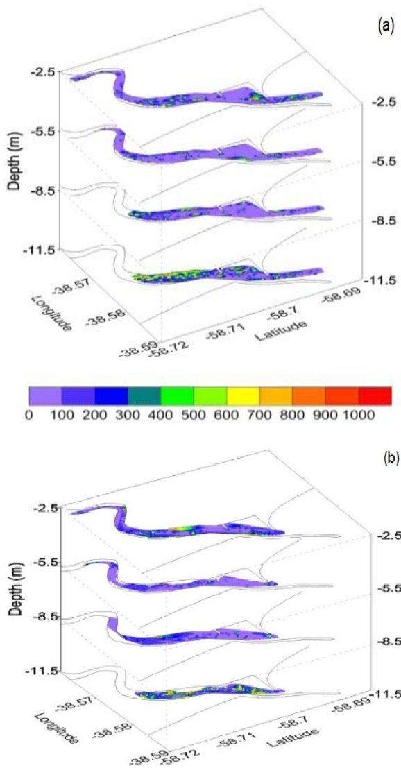
Figura 2: Distribución de los valores de S_A (en m^2/min^2 ) integrados en estratos de 3m durante el (a) flujo y (b) reflujos en un estuario mezclados.
