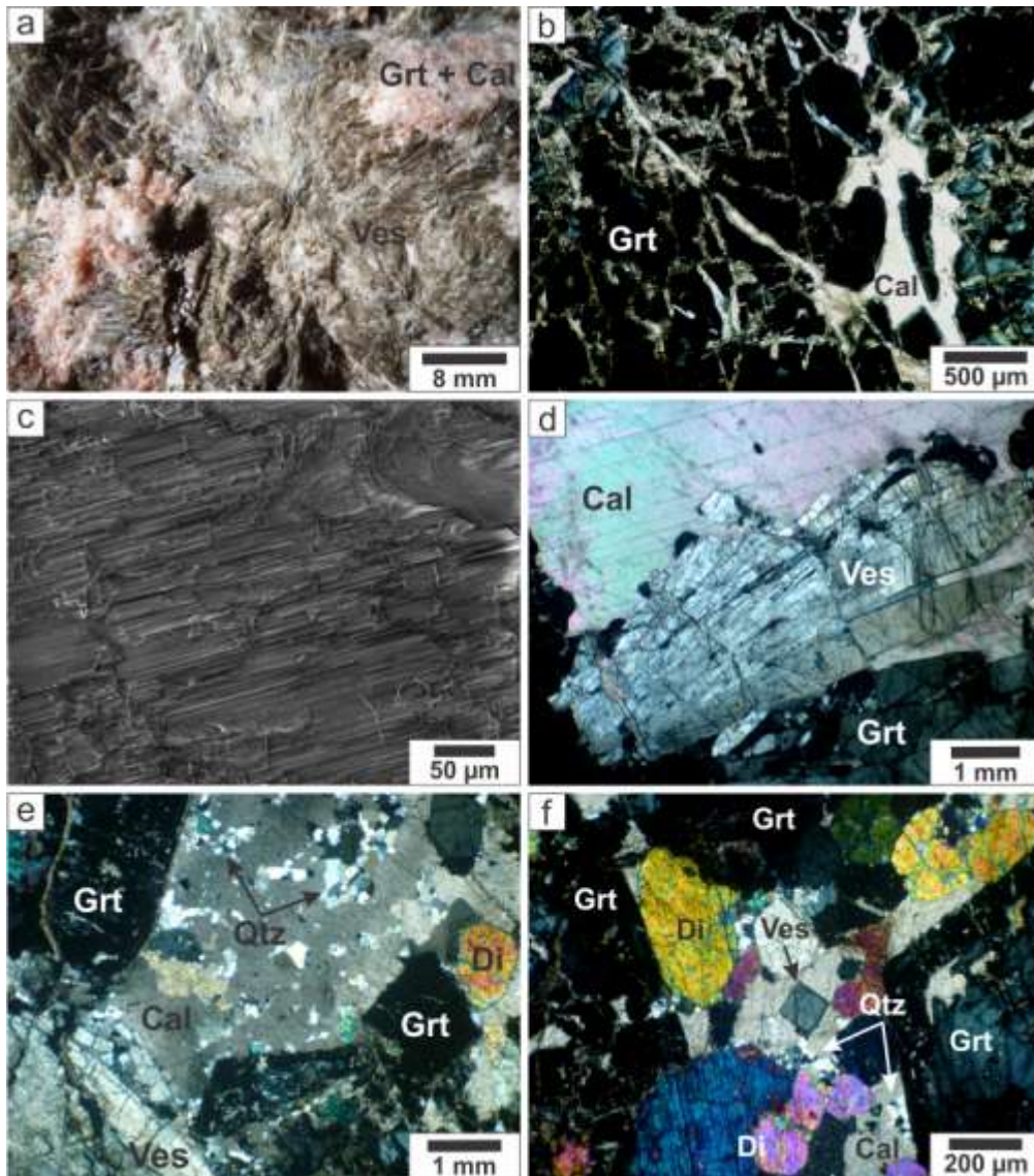
Figura 2. a) “Soles” de vesuvianita (Ves) en muestra de mano (LM-13). b) Base granatífera craquelada con calcita (Cal) relleno microfracturas [LM-13; con analizador (LPA)]. c) Estrías en la superficie de un cristal de Ves visto con microscopio electrónico de barrido. d) Agregado radial de cristales de Ves (LM-13; LPA). e) Grt, Ves y diópsido (Di) en matriz de Cal y presencia de mosaicos de cuarzo (Qtz) (LM-9; LPA). f) Ves (sección basal) en asociación con Grt y Di en matriz de Cal (LM-9; LPA). Abreviaturas de los minerales según Kretz (1983).
