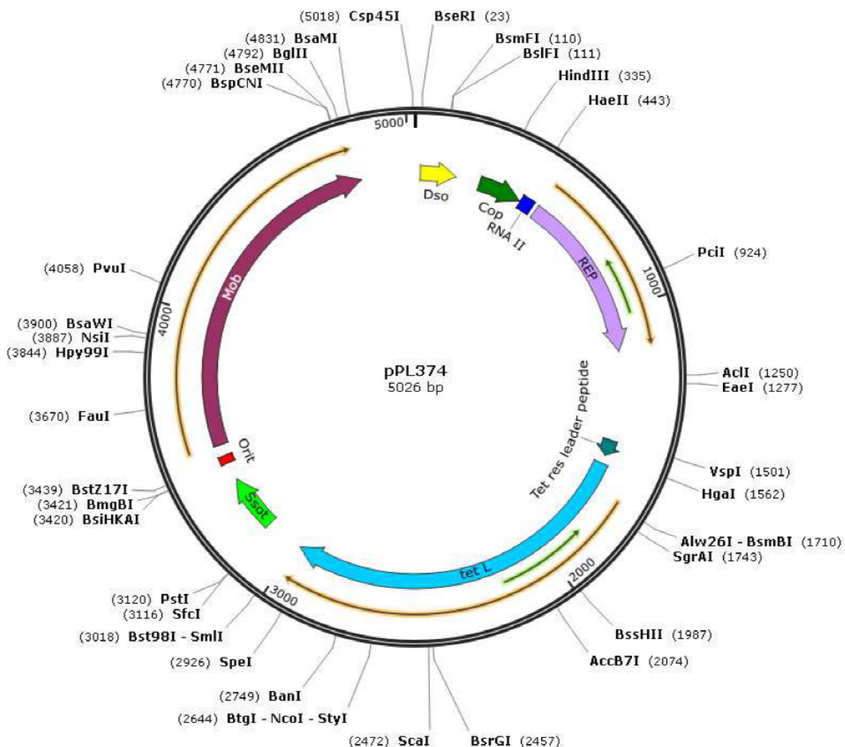
Figura 57: Representación esquemática del plásmido pPL374 aislado de la cepa de Paenibacillus larvae PL374 con resistencia a tetraciclina y oxitetraciclina. Los elementos se asignaron de acuerdo con la homología encontrada con otros elementos de plásmidos conocidos: dso : Origen de replicación de doble hebra; Cop : Represor transcripcional (gen Cop ), RNA II : ARN contra transcrito; rep : Inicio de replicación; tetL : Gen de resistencia a tetraciclina por eflujo activo; sso : Origen de replicación de simple hebra; mob : Función de movilización (gen mob ) y oriT : Origen de transferencia. Las flechas más externas (amarillas y verdes) indican la dirección de los marcos de lectura abierta (traducción mínima de 75 aminoácidos). Se señalan también los sitios de corte de distintas enzimas de restricción.
