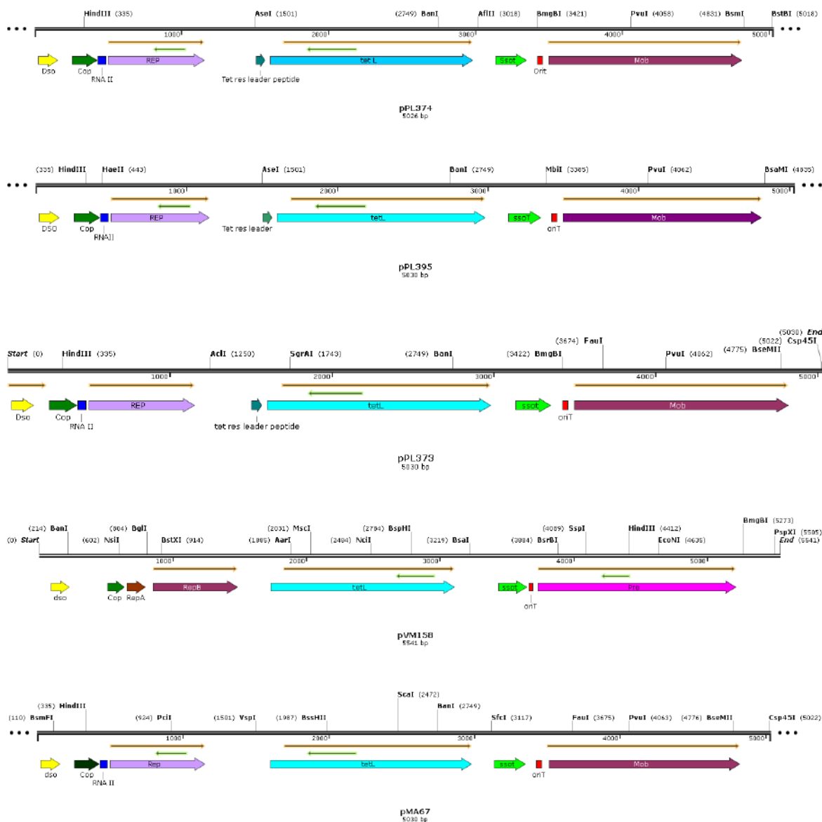
Figura 58: Comparación esquemática de los plásmidos pL374, pL395 y pL373 con el plásmido pM158 de Streptococcus agalactiae y pMA67 de Paenibacillus larvae . Los elementos se asignaron de acuerdo con la homología encontrada con otros elementos de plásmidos conocidos: dso : Origen de replicación de doble hebra; Cop : Represor transcripcional (gen Cop ), RNA II : ARN contra transcrito, rep : Inicio de replicación; tetL : Gen de resistencia a tetraciclina por eflujo activo; sso : Origen de replicación de simple hebra; mob : Función de movilización (gen mob ) y oriT : Origen de transferencia. Se indican los marcos de lectura abierta de traducción de un mínimo de 75 aminoácidos y que comienzan con el codón ATG.
