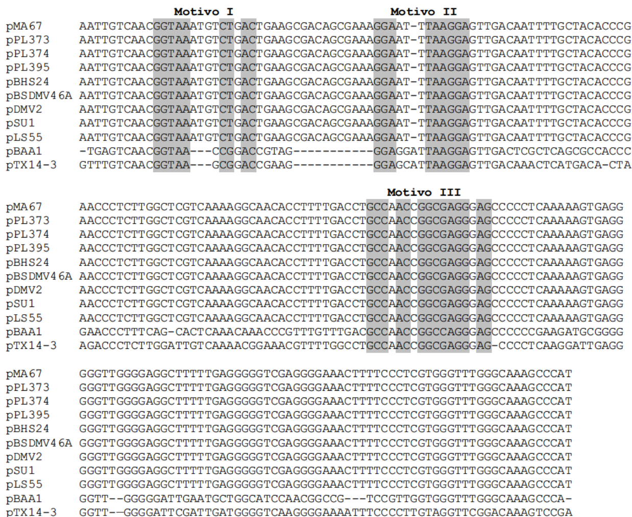
Figura 60: Alineamiento de las secuencias del origen de replicación simple hebra ( ssu ) de los plásmidos pPL373, pPL374 y pPL395 en comparación con otros plásmidos de tipo ssuT dentro de los que se replican por el mecanismo de círculo rodante. Los plásmidos usados en la comparación fueron: pMA67 ( Paenibacillus larvae ), pBHS24 ( Bacillus sp.), pBSDMV46A ( Barghavaea cecembensis ), pDMV2 ( Bacillus galactosidilyticus ), pSU1 ( Sporosarcina ureae ), pLS55 ( Lactobacillus sakei ), pBAA1 ( Bacillus spp.) y pTX14-3 ( Bacillus thuringiensis serovar israelensis ). Se marcan las posiciones de los tres motivos (I, II y III) en distintos tonos de sombreado.
