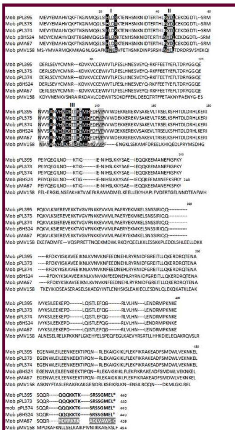
Figura 61: Alineamiento de las secuencias de aminoácidos de las proteínas Mob de los plásmidos de Paenibacillus larvae pPL395, pPL373, pPL374, pBHS24 ( Bacillus sp.) y pMA67 ( P. larvae ) en comparación con el plásmido pMV158 de Streptococcus agalactiae . Sólo se representa el plásmido pBHS24 no obstante, las secuencias de las proteínas Mob son idénticas a las de los plásmidos pBSDMV46A ( Barghavaea cecembensis ), pDMV2 ( Bacillus galactosidilyticus ), pSU1 ( Sporosarcina ureae ), pAST4 (bacteria marina no cultivable) y pLS55 ( Lactobacillus sakei ). En subrayado se indican los motivos conservados (I, II y III) de la familia MOBV; en letras blancas y fondo negro se indican los aminoácidos invariables, en letras negras y gris claro se indican los aminoácidos altamente conservados dentro de la superfamilia pMV158. En letras blancas y gris oscuro se marcan las diferencias con el plásmido pMA67 lo que genera dos relaxasas diferentes en el N terminal.
