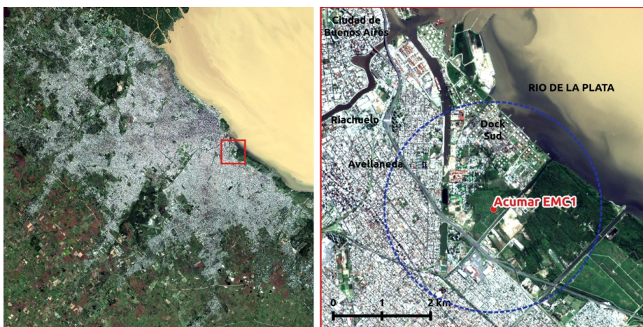
Figura 1. Región Metropolitana de Buenos Aires (izquierda) y ubicación de la Estación de Monitoreo Continuo y Automático de la Calidad del Aire en Dock Sud (EMC I) (derecha). El círculo azul indica el área de influencia de la estación. Fuente: Imagen Sentinel-2 (ESA) 14 de abril del 2017.
