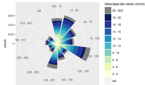
Figura 2. Rosa de los vientos para el período 01/01/2011 - 30/10/2016
