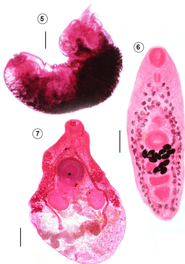
FIGURES 5-7. Digeneans from P. brasiliensis . 5. Strigea falconis brasiliensis . Bar = 200 µm. 6. Ribeiroia ondatrae . Bar = 200 µm. 7. Prosthogonimus ovatus . Bar = 500 µm.
