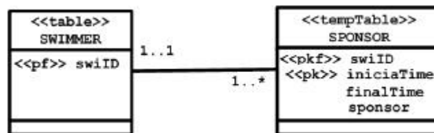
Gráfico 6. Transformación del atributo temporal a UML
