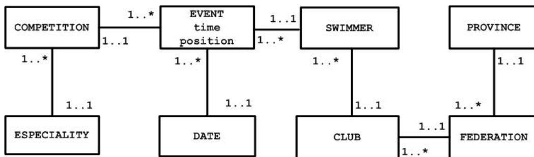
Gráfico 2. Esquema copo de nieve
