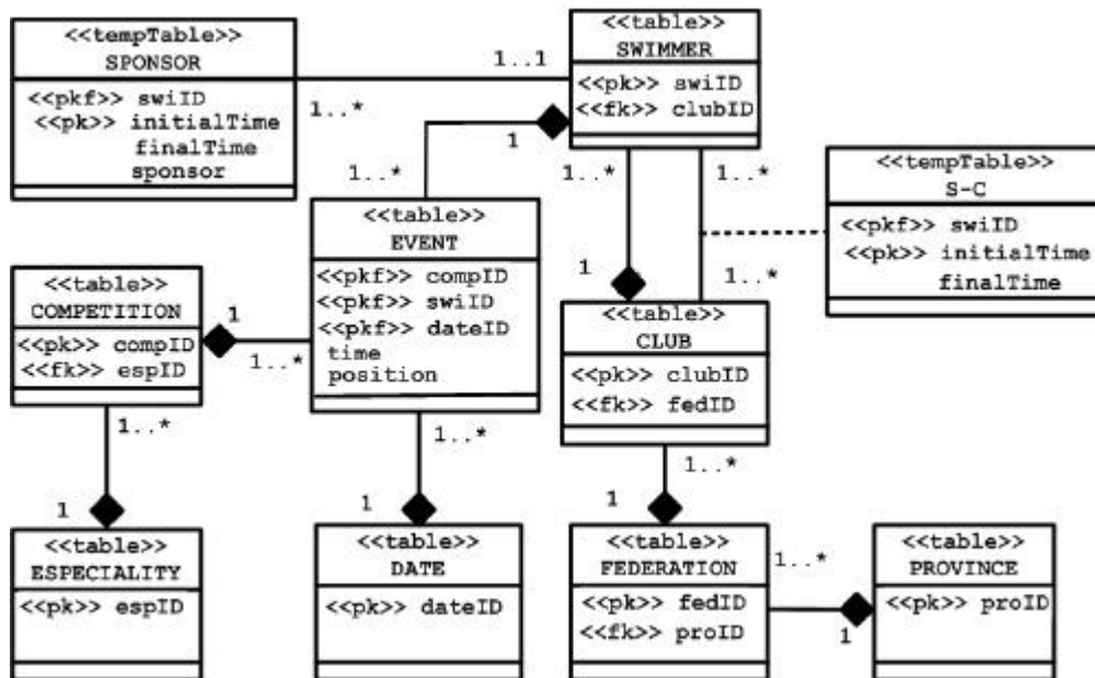
Gráfico 10. Transformación del esquema multidimensional temporal a UML
