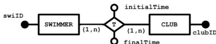
Gráfico 7. Interrelación temporal
