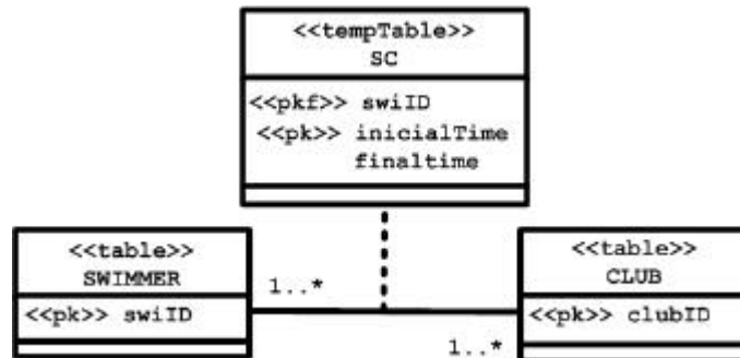
Gráfico 8. Trasformación de la interrelación temporal a UML
