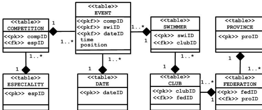
Gráfico 3. Transformación del esquema copo de nieve a UML
