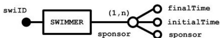
Gráfico 4. Atributo compuesto multivaluado
