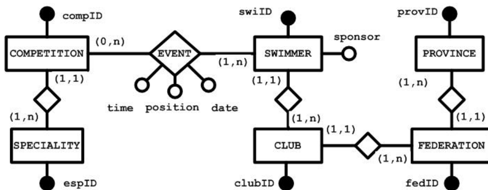
Gráfico 1. Diagrama entidad-interrelación
