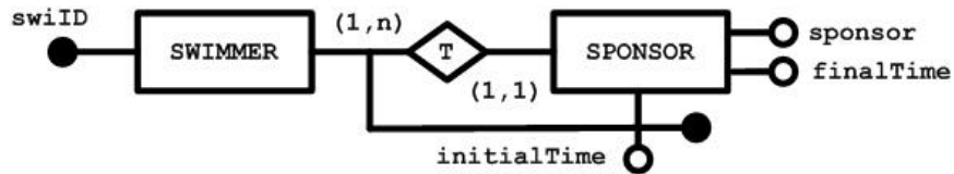
Gráfico 5. Transformación de atributo temporal
