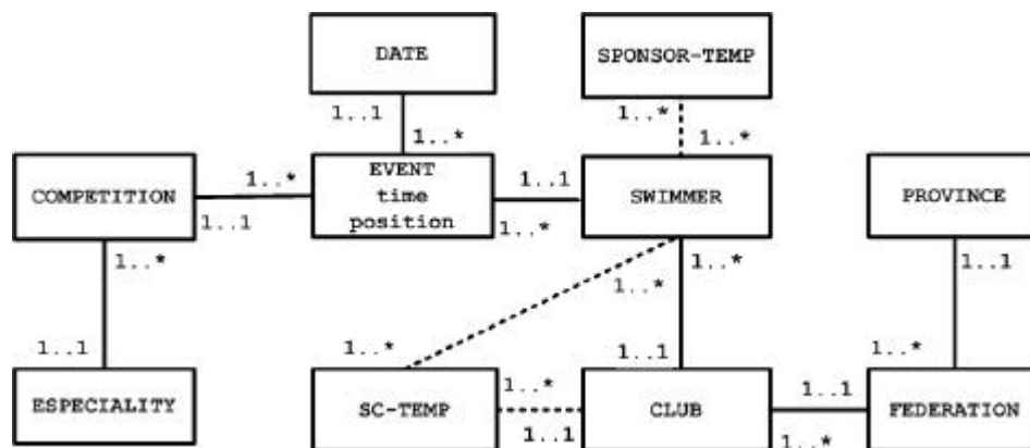
Gráfico 9. Esquema multidimensional temporal
