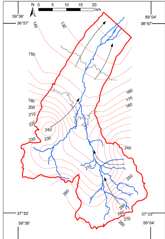
Fig. 3. Mapa equipotencial de la cuenca del arroyo Chapaleofú para noviembre de 2019.
