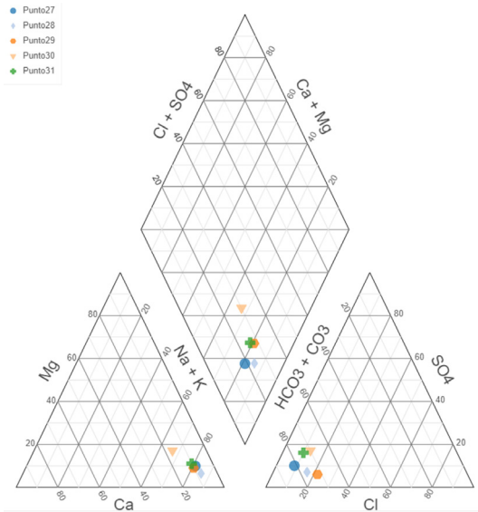
Fig. 8. Diagrama de Piper para la zona de llanura de la cuenca (según datos de noviembre de 2019).
