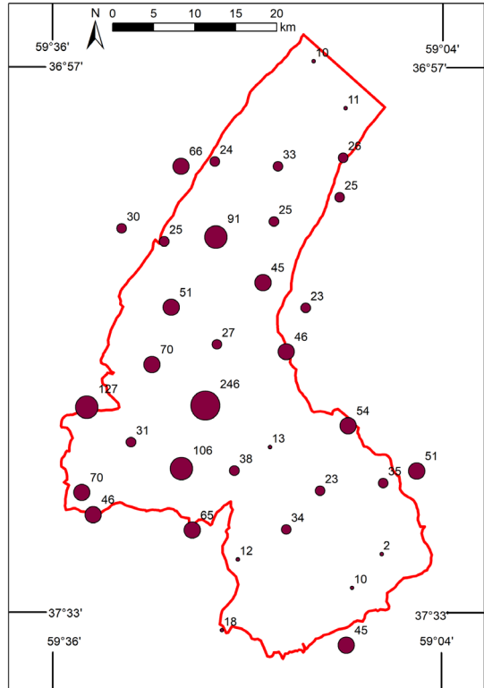
Fig. 9. Distribución espacial de los nitratos en la cuenca del arroyo Chapaleofú para noviembre de 2019.
