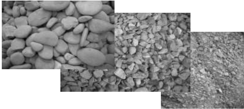
Foto 6 - Paso de un canto rodado de 4 pulgadas a árido 6:20 y arena de trituración 0:6 con el sistema descripto
