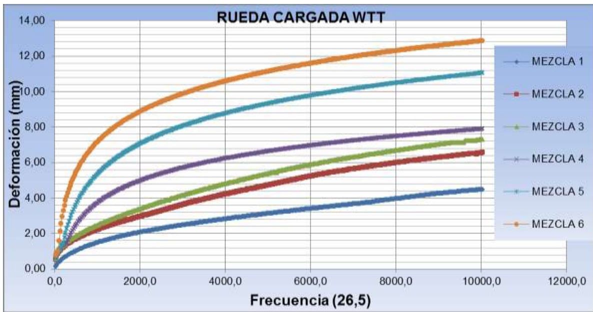
Gráfico 1 - Curvas de deformación y frecuencia
