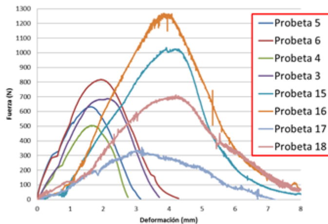
FIGURA 18 Curvas centrales; moldeo manual.
