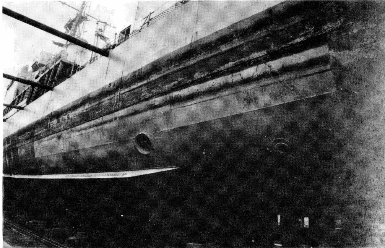
Figura 8.- Vista panorámica del costado babor de una embarcación, donde puede observarse la efectividad de diferentes pinturas antiincrustantes después de quince meses de inmersión
