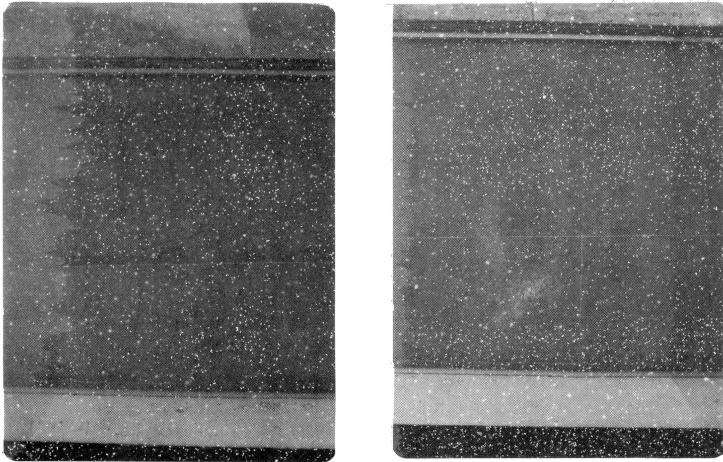
Fig. 9.- Paneles correspondientes a las pinturas nº 7 y nº 8, formuladas con óxido cuproso, arseniato mercurioso y carbonato de calcio, aplicadas sobre el costado babor del Crucero ARA General Belgrano, luego de 12 meses de inmersión
