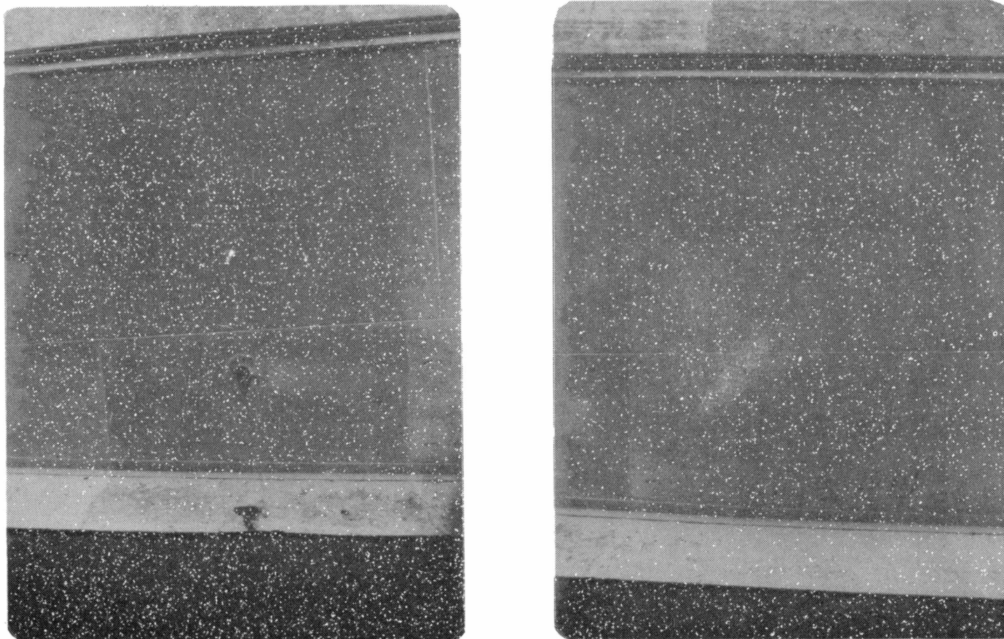
Fig. 8.- Paneles correspondientes a las pinturas nº 5 y nº 6, formuladas con óxido cuproso y arseniato mercurioso, aplicadas sobre el costado babor del Crucero ARA General Belgrano, luego de 12 meses de inmersión
