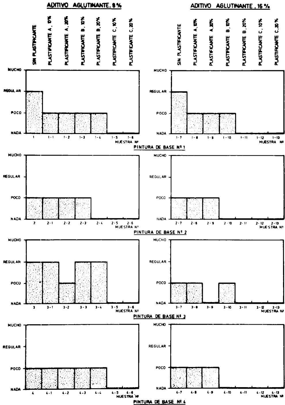
FIGURA Nº 2 - ENSAYO DE ENVEJECIMIENTO ACCELERADO - EXPOSICION EN WEATHER OMMETER SUNSHINE ARC XW - 700 horas - CUARTEADO
