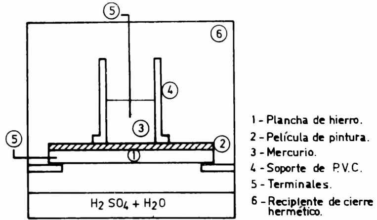
FIGURA 9 - MEDIDAS DE RESISTENCIA Y CAPACIDAD EN EL AIRE.
