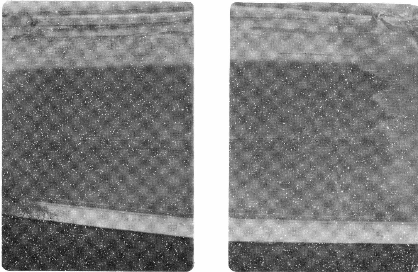
Fig. 7.- Paneles correspondientes a las pinturas nº 2 (formulada con óxido cuproso, izquierda) y nº 3 (con óxido cuproso e inertes, derecha) aplicadas sobre el costado babor del Crucero ARA General Belgrano luego de 12 meses de inmersión
