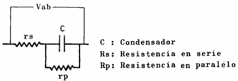
FIGURA 6 - CIRCUITO EQUIVALENTE.
