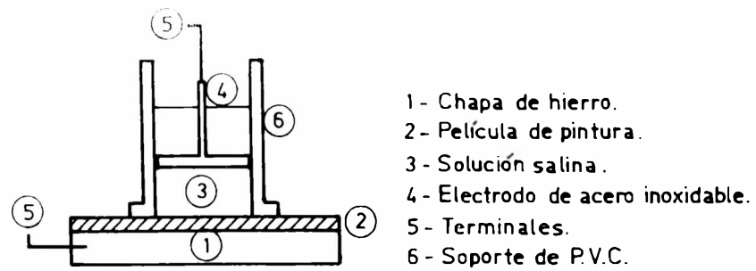
FIGURA 10 - MEDIDAS DE RESISTENCIA Y CAPACIDAD EN AGUA.
