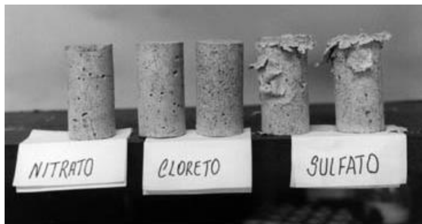
Figura 1: Visão geral dos corpos de prova à base de cal e areia, após uma sobrecarga de sais higroscópicos. Fonte: Nappi [1]
