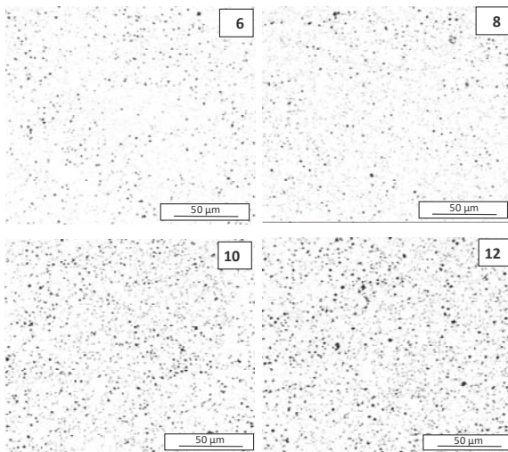
Fig. 2 Imágenes electrónicas de cada condición y distribución de TiC.
