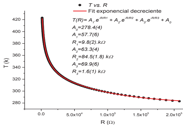
Figura 6: Curva empírica de la temperatura T del cubo vs. La resistencia R del termistor. En rojo se representa una función suma de exponenciales decrecientes utilizada para ajustar una curva a los datos.
