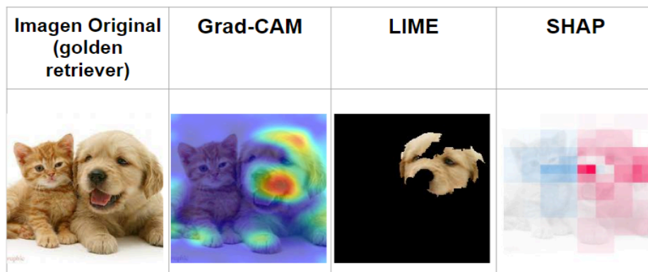
Fig. 1. Resultados de aplicar los métodos de visualización Grad-CAM, LIME y SHAP sobre la clasificación de una imagen mediante una red neuronal convolucional
