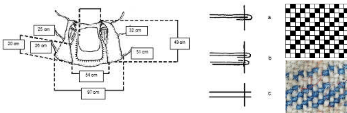
Figura 4. De la izquierda hacia la derecha: Esquemas con las dimensiones del chaleco; representación de la disposición de las telas en relación a las puntadas y fotografía de los ligamentos de la tejido de algodón acompañada de su representación gráfica.
