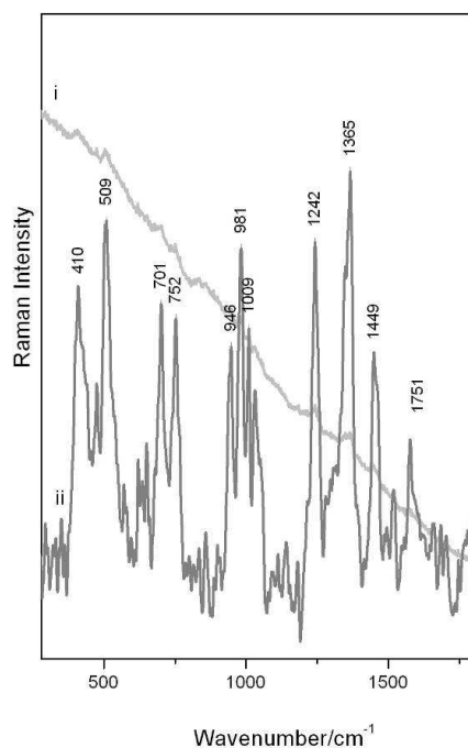
Figura 6. Espectro de tela teñida de rojo por i) Raman convencional y ii) SERS con corrección de la línea de base. Fuente: Center SMAArt - Scientific Methodologies applied to Archaeology and Art.
