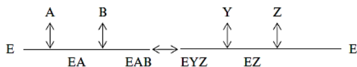
Figura 2.6. Mecanismo secuencial ordenado [8].
