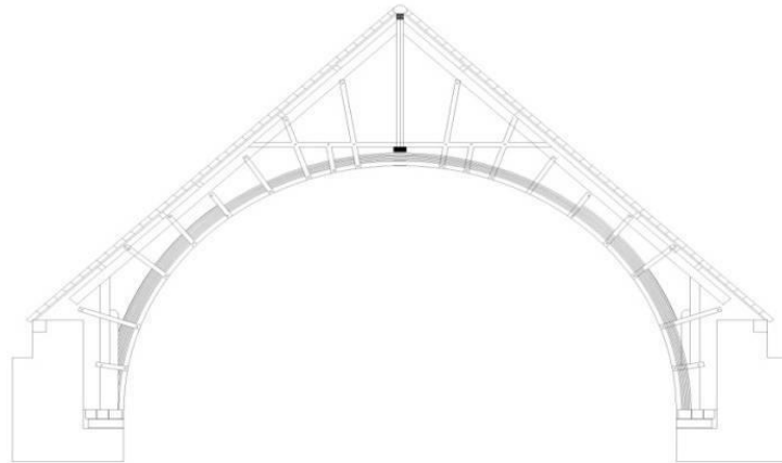
Fig. 6. Estructura de Madera. Francisco Méndez Flores.
