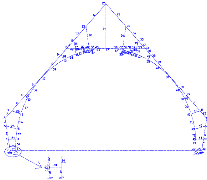
Fig. 7. Estructura de Madera, Francisco Méndez Flores.
