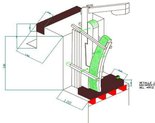
Fig. 8 Disposición de la estructura de madera mostrando aisladores del tipo elástico. Francisco Méndez Flores.
