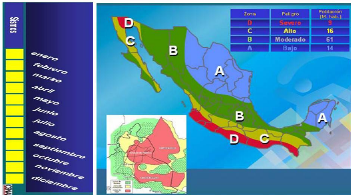
Fig. 2 regionalización sísmica de la República Mexicana.
