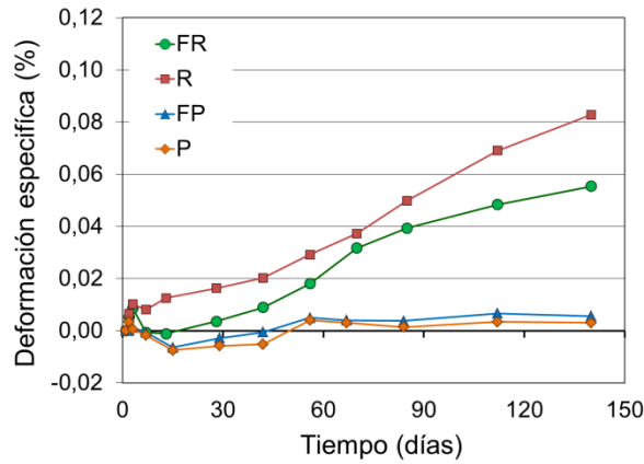
Figura 3. Variaciones dimensionales en prismas de 70x70x300 mm.
